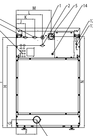
Zadní pohled
